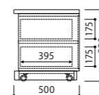
抽斗ボックス D50-H55
