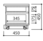
抽斗ボックス D45-H45
