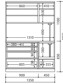
SDH-4183SK-42-C-D45 正面図
