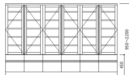
SDF-4556-HK45 下段抽斗レール付 +¥132,000 (¥120,000)
