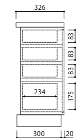
抽斗ボックス D33
