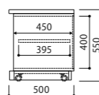
扉ボックス D50-H55
