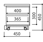
扉ボックス D45-H45
