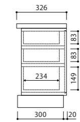
抽斗ボックス D33
