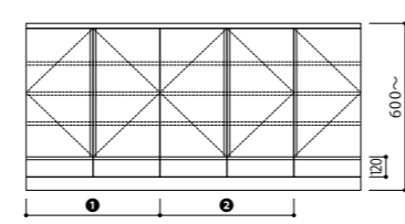
SDF-4555L-G10 最下段抽斗付 +¥44,000 (¥40,000) ※ 抽斗レールは付きません
