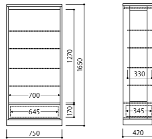
SDH-R4502-CB (観音開き)
