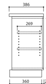
扉ボックス D40
