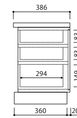
抽斗ボックス D40
