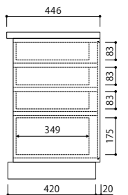
抽斗ボックス D45
