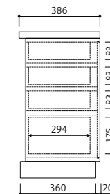
抽斗ボックス D40
