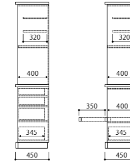
SDH-4183SK-42-C-D45 側面図
