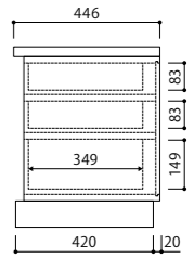
抽斗ボックス D45
