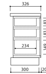
抽斗ボックス D33
