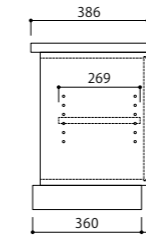
扉ボックス D40
